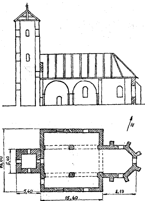
Figura 10. Șard; plan și secțiune longitudinală după V. Brătulescu
