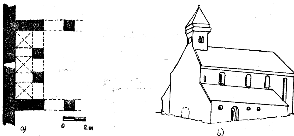
Figura 5. Gîrbova; plan (a) și reconstituire (b), după W. Horwath
