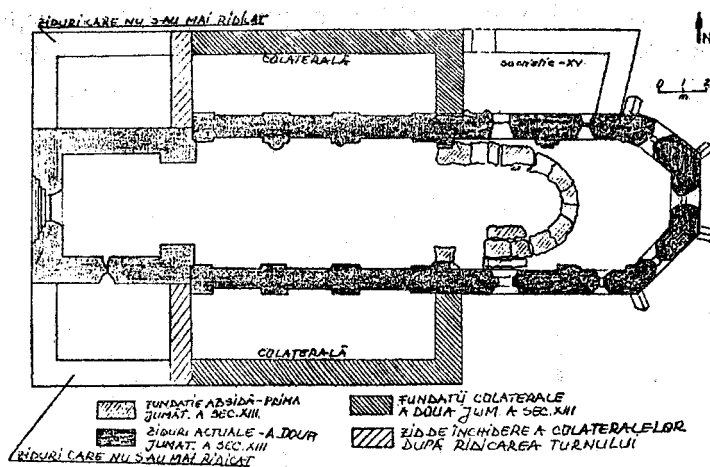
Figura 4. Cricău; plan după R. Heitel
