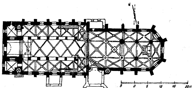
Figura 9. Sebeș; plan după V. Vătășianu
