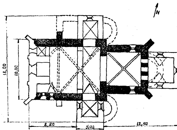
Figura 11. Vințu de Jos; plan după I. Șerban
