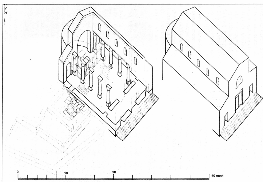
Fig. 2. Reconstituire axiometrică a basilicii „Florescu” (arh. I. Baldescu, în Histria - ghid album )
