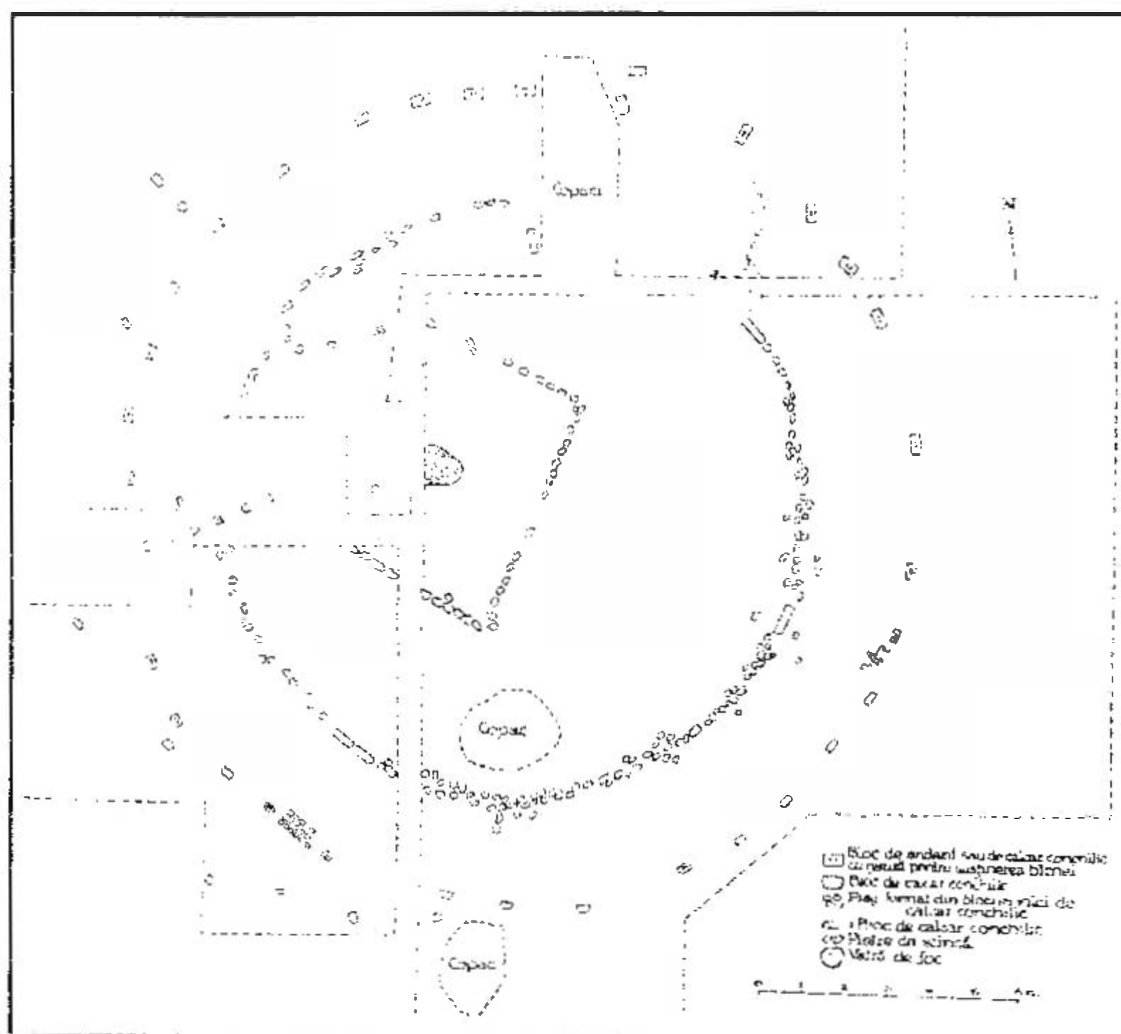
Fig. 2. Planul locuinței de pe dealul Pustâiosu (după C. Daicoviciu și colab.)
