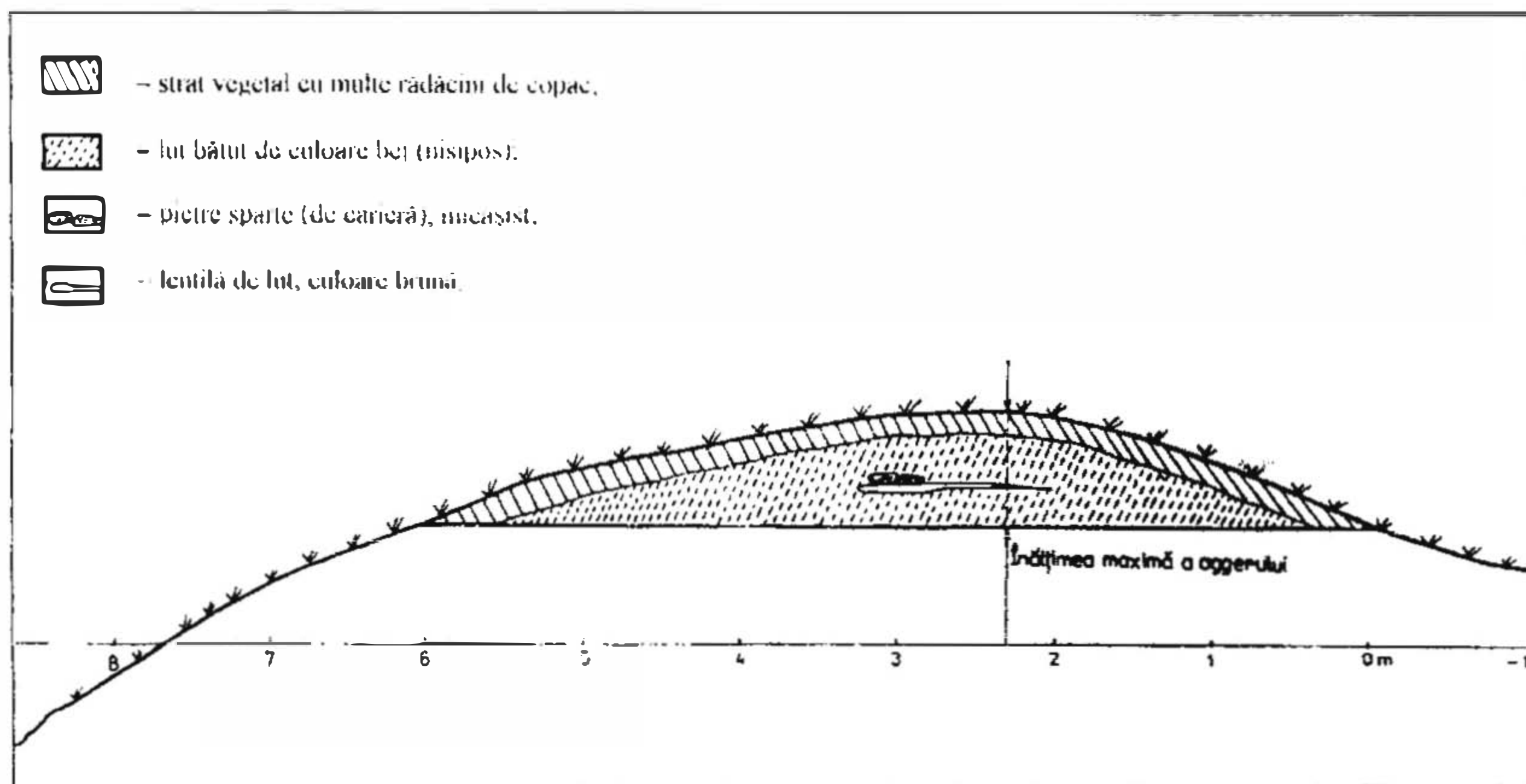
Fig. 2. Structura și forma agger -ului sudic al fortificației romane de la Cornuțel.
