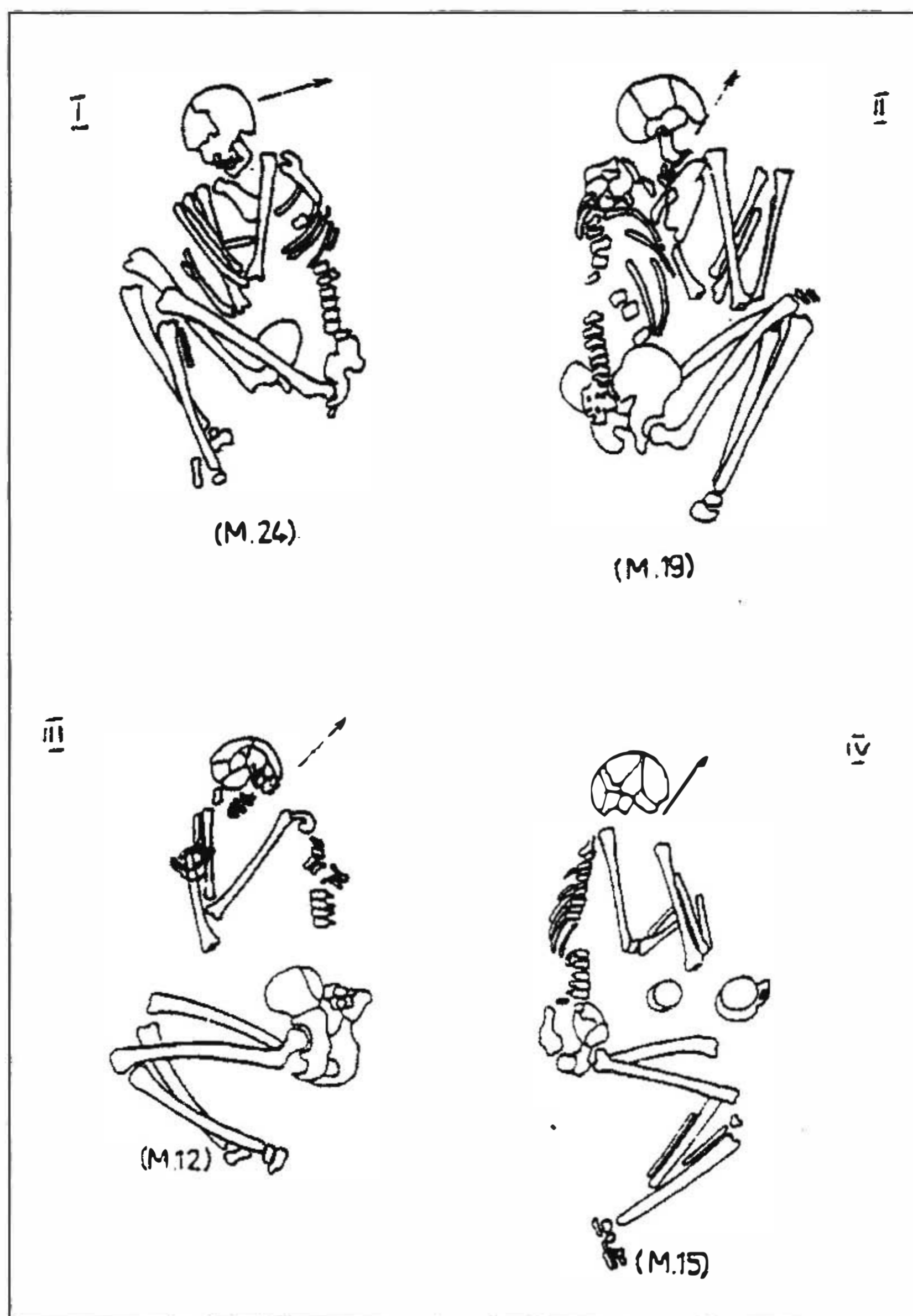
Fig. 3. Grade de chircire a scheletelor: de la chircit foarte accentuat (I) către chircit moderat (IV)
